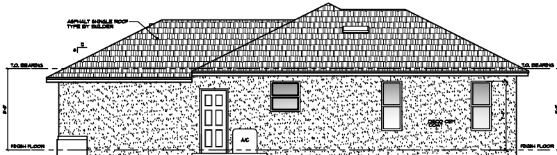
RIGHT ELEVATION SCALE: 1/4"=1'-0"
